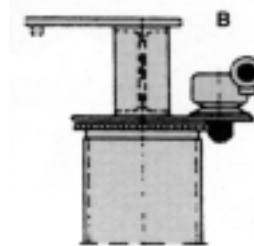
Typ B för utomhusbruk och utligg mer än 8 meter. Drivning sker med kuggkran.
